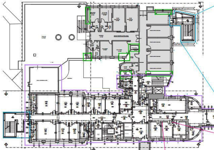
PROGETTO ARCHITETTONICO Pianta Piano Primo
