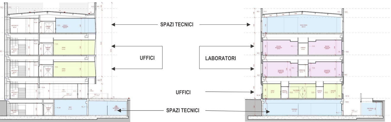
SEZIONE A
